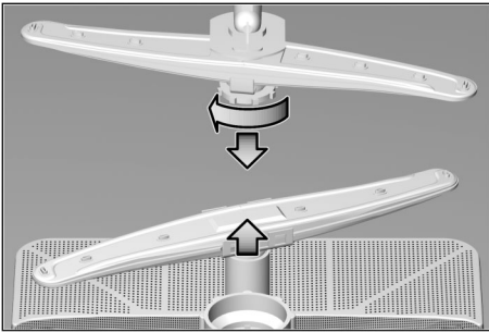
Bras pivotants
