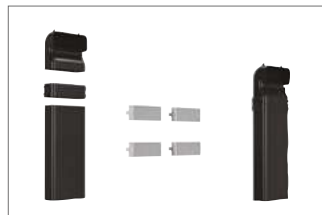
HEZ9VDKE1 montážní sada pro odtah pro varné desky s odsáváním, pro hloubku pracovní desky 60 cm a větší (4x akustické filtry, 1x ploché vertikální koleno 90° "S", 1x plochý spojovací díl, 1x ploché potrubí 50 cm) Cena: 3 490 Kč*
