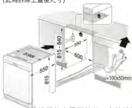
櫥櫃安裝示意圖 (此為折除上蓋後尺寸)
