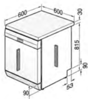
產品尺寸圖 (此為獨立安裝尺寸)
