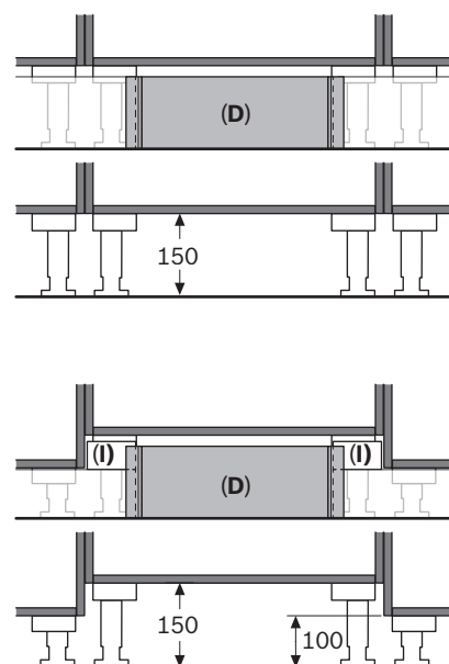
Rozměry v mm Varianty soklu pro robotický modul
