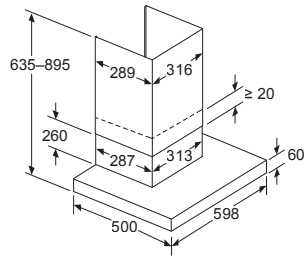
Apparecchio in modalità di estrazione dell'aria
