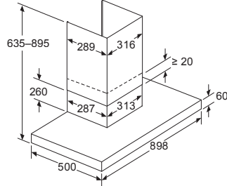
Apparecchio in modalità di estrazione dell'aria
