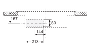
Vorderansicht - Möbelausschnitt für Umluft ohne Kanal
