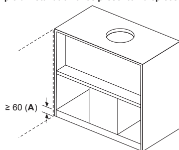
Exemple d'installation avec présentoir à épices
