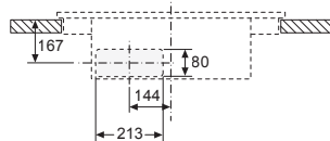
Vue de face - découpe du meuble pour circulation d'air sans conduit
