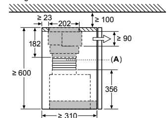
Montage Clean Air Modul mit integrierter Designhaube
