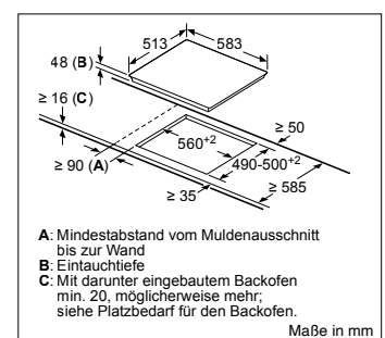
PKN645FP2E – umlaufender Rahmen
