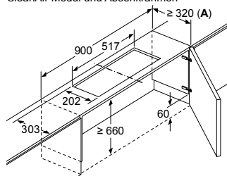
Montage Flachschrümhaube mit CleanAir Modul und Absenkrahmen
