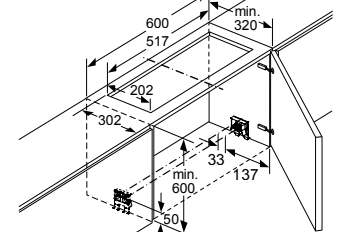
Montage Flachschrümhaube mit Clean Air Modul
