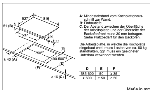
PXY875DW4E, PXY875DC1E – Comfort Profil
