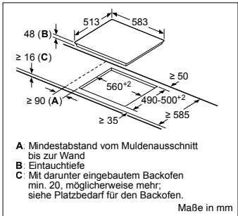
PKE645BA2E – umlaufender Rahmen
