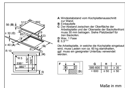
PXV901DV1E – flächenbündig
