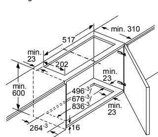
Montage Lüfterbaustein mit Clean Air Modul
