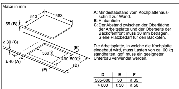
NXX645CB5E | NVS645CB6E – umlaufender Edelstahl-Rahmen
