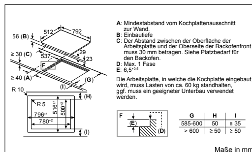
PXY801DW4E – flächenbündig
