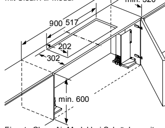
Montage Flachschrümhaube mit Clean Air Modul
