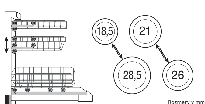
Systém košov s 3. košom Extra Space pri umývačkách s výškou 81,5 cm
