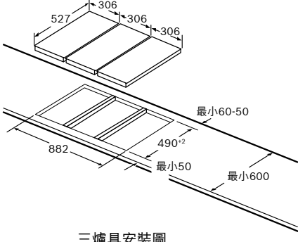
三爐具安裝圖
