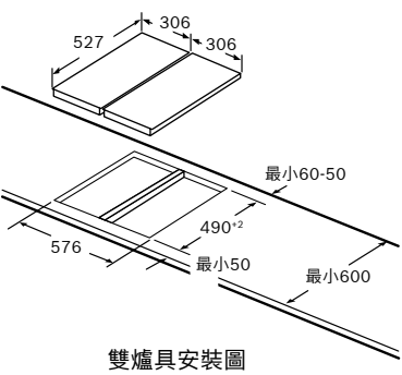
雙爐具安裝圖
