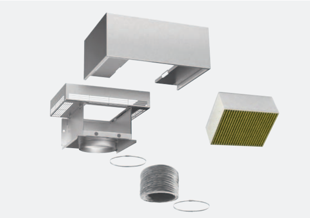
Esempio: modulo a ricircolo Clean Air Plus esterno con pannello di design per montaggio a parete e sul canale.
