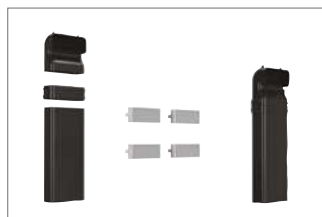
HEZ9VDKE1 montážní sada pro odťah pro varné desky s odsáváním, pro hloubku pracovní desky 60 cm a větší (4x akustické filtry, 1x ploché vertikální koleno 90° "S", 1x plochý spojovací díl, 1x ploché potrubí 50 cm) Cena: 3 490 Kč*
