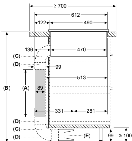
Kringloopwerking met afvoerkanalen tot onder meubel/plint – werkbladdiepte ≥ 700 mm
