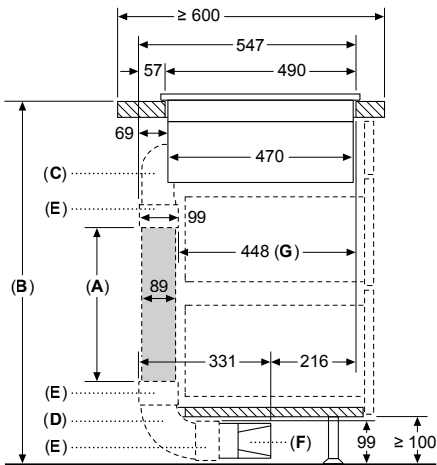
Kringloopwerking met afvoerkanalen tot onder meubel/plint – werkbladdiepte ≥ 600 mm
