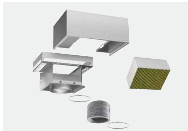
Príklad: montážna súprava pre nástenný odsávač pár s prevádzkou cirkulácie s filtrom CleanAir Plus
