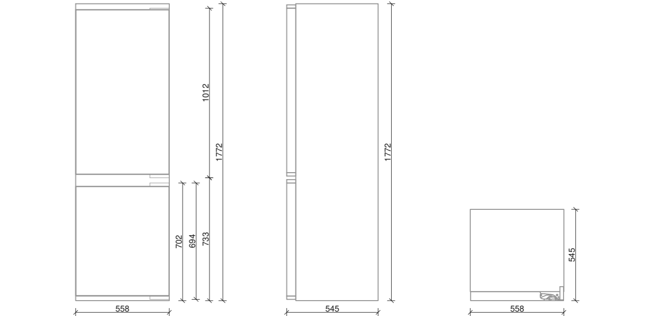
BOSCH KIN86AF31K
