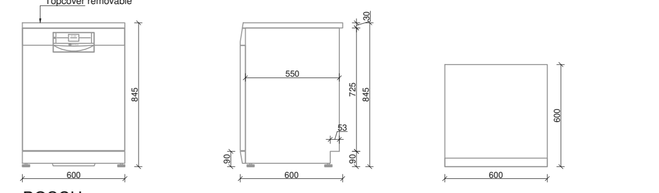
BOSCH SMS8YCI01E
