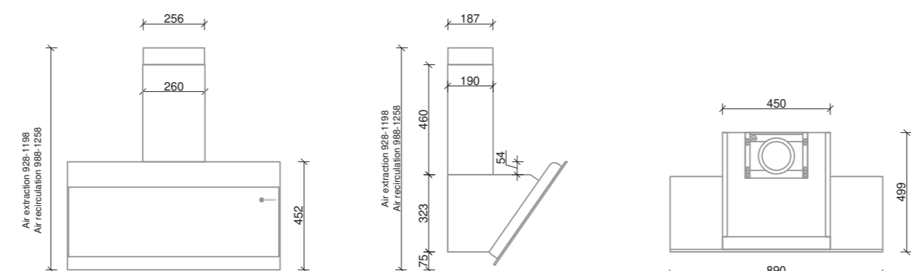
BOSCH DWK97JM20
