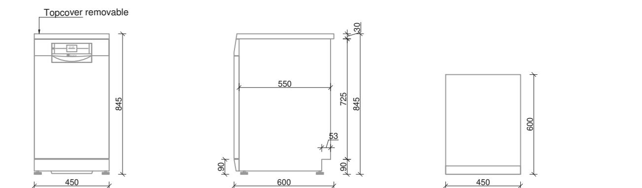
BOSCH SPS6ZMI35E
