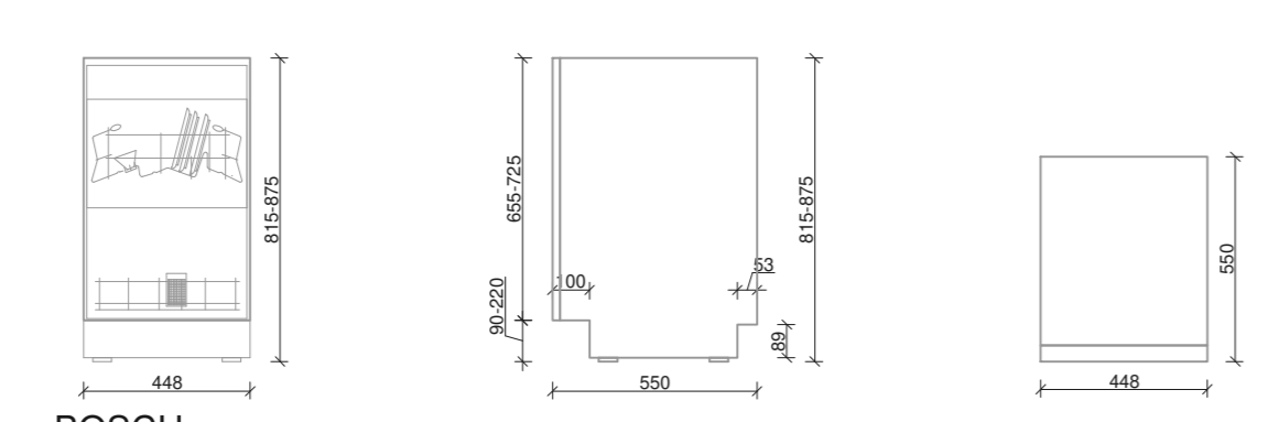
BOSCH SPV4XMX28E
