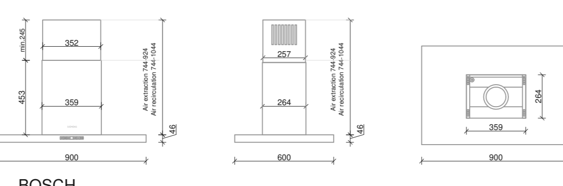
BOSCH DIB98JQ50B
