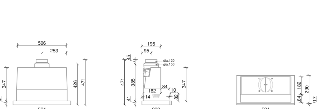
BOSCH DFS067A51B
