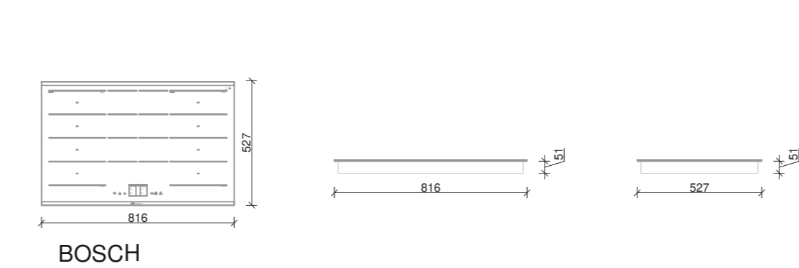
BOSCH PXY875KW1E
