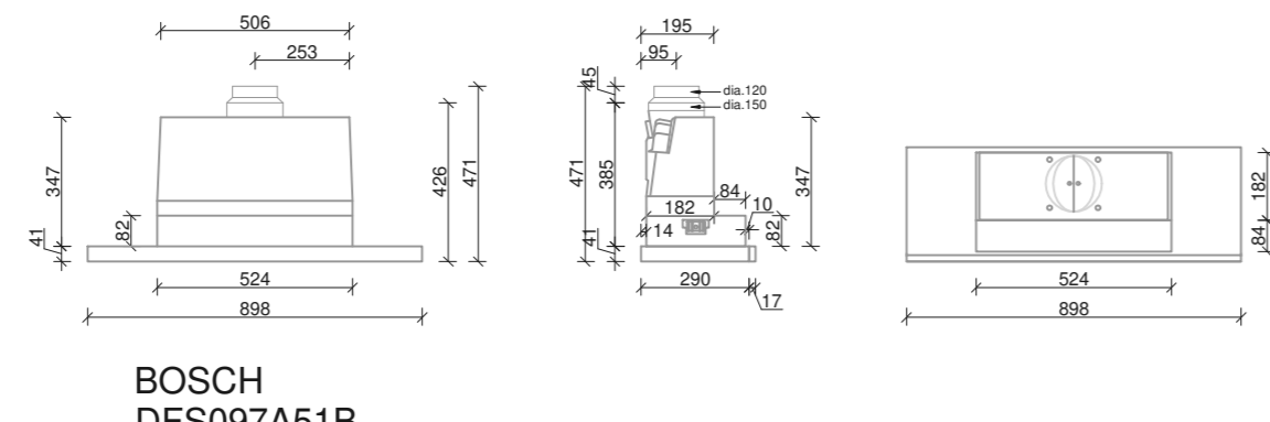
BOSCH DFS097A51B
