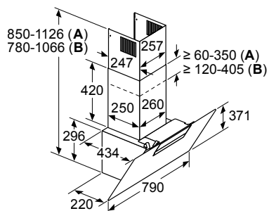
A: Circulatielucht B: Luchtafvoer - sleuf naar onderen gericht monteren
