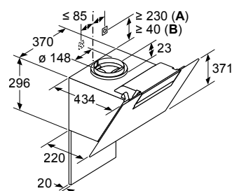
A: Geïntegreerde Clean Air B: Luchtafvoer of standaard circulatieluchtset Rekening houden met de maximale dikte van de achterwand.
