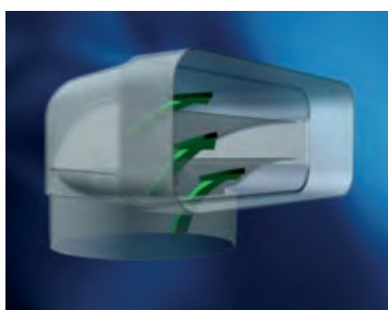
Nové potrubní systémy s integrovanými prvky vedení vzduchu
