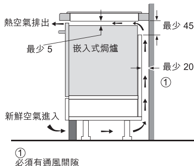
電磁爐安裝在焗爐上方
