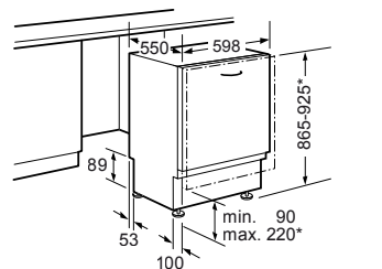
Afmetingen in mm
