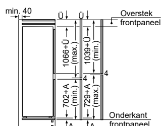
De aangegeven meubeldeurmatten gelden voor een deurnaad van 4 mm. Afmeting in mm
