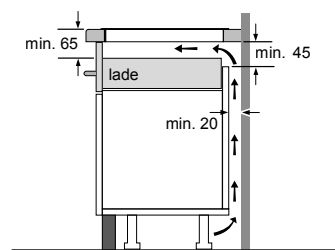
Afmetingen in mm
