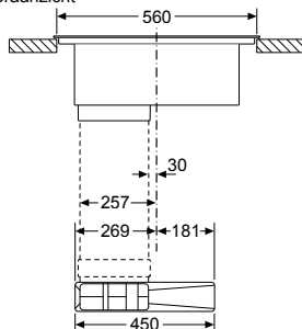
Afmetingen in mm Vooraanzicht
