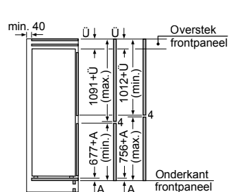
De aangegeven meubeldeurmatten gelden voor een deurnaad van 4 mm. Afmeting in mm
