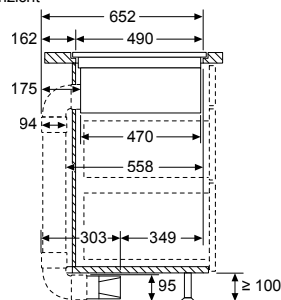
Afmetingen in mm Zijaanzicht
