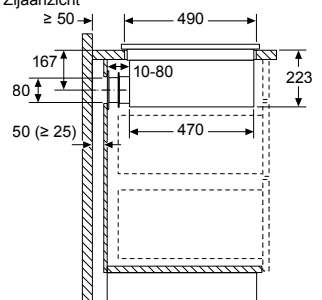
Afmetingen in mm Zijaanzicht
