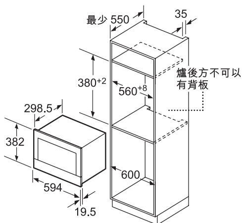
微波爐設於高櫃
