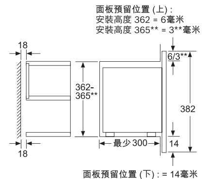
微波爐面板上下預留位置
