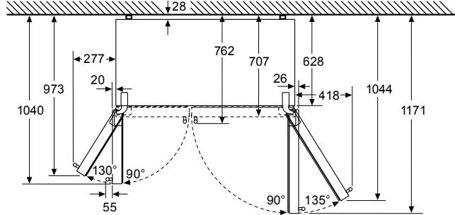
Afmeting in mm
