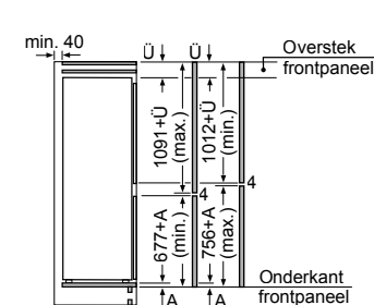
De aangegeven meubeldeurmatten gelden voor een deurmaad van 4 mm. Afmeting in mm
