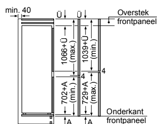
De aangegeven meubeldeurmatten gelden voor een deurmaad van 4 mm. Afmeting in mm
