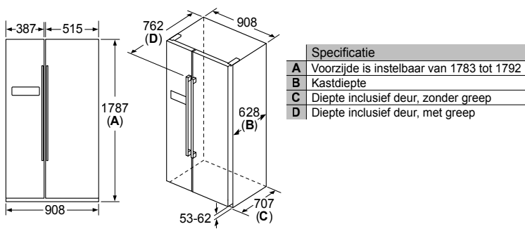
Afmeting in mm
