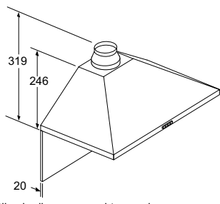
Bij gebruik van een achterwand moet met het design van het apparaat rekening worden gehouden. Afmeting in mm
