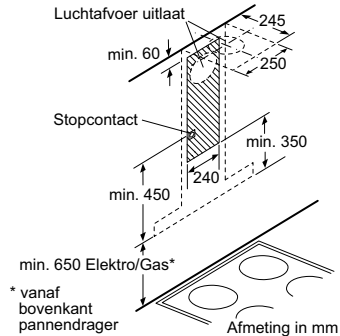
min. 650 Elektro/Gas* * vanaf bovenkant pannendrager
