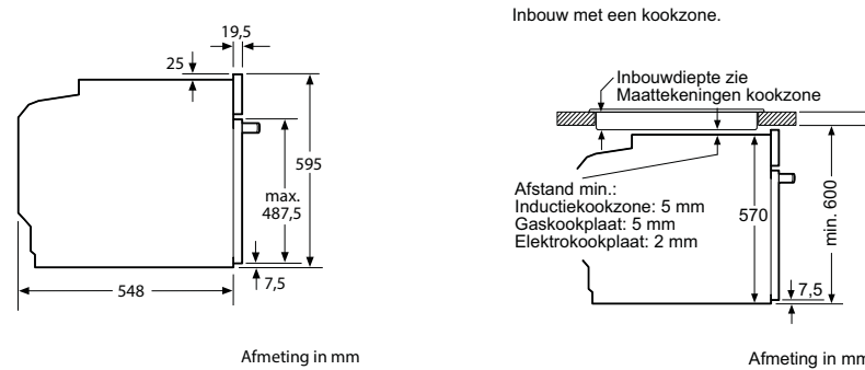
Inbouw met een kookzone.
