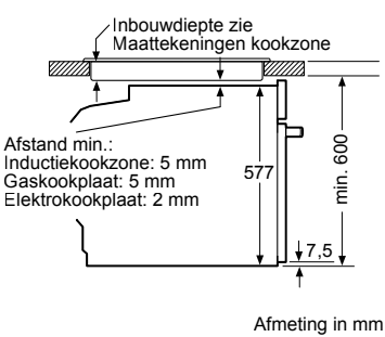
Inbouw met een kookzone.
