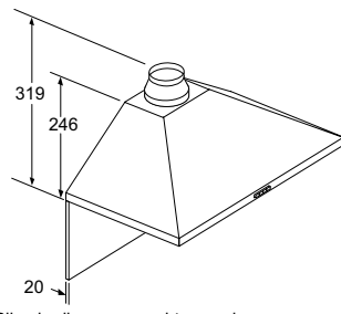
Bij gebruik van een achterwand moet met het design van het apparaat rekening worden gehouden. Afmeting in mm
