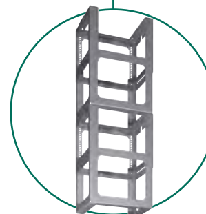
Extension de 1 mètre pour kit de montage (nécessaire pour l'installation d'une extension de cheminée de 1,6 mètre). DHZ1253 Code barre : 4242002510231 Compatible avec : DIB97IM50
