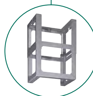
Extension de 0,5 mètre pour kit de montage (nécessaire pour l'installation d'une extension de cheminée de 1,1 mètre). DHZ1251 Code barre : 4242002510217 Compatible avec : DIB97IM50
