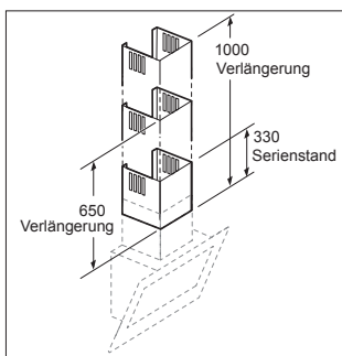
DUL63CC50 | DUL63CC20 | DUL63CC40 | DUL62FA51 | DUL62FA21
