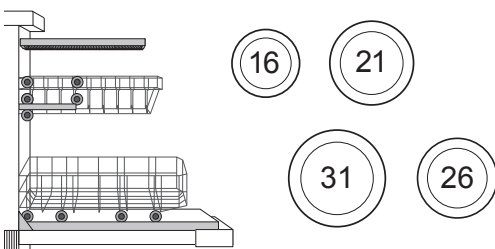
Korbssystem mit VarioSchublade Gerätehöhe 81,5 cm
