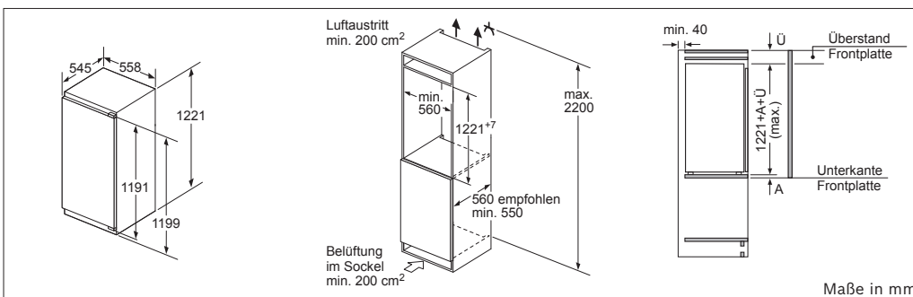
KIF ... | KIR41A ... | KIL42A ...
