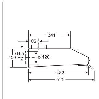
DUL63CC50 | DUL63CC20 | DUL63CC40 | DUL62FA51 | DUL62FA21
