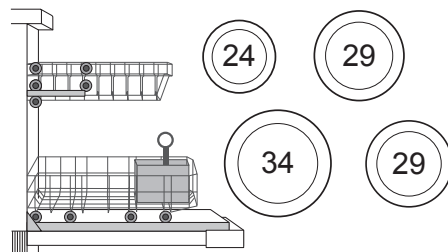
Korbssystem ohne VarioSchublade Gerätehöhe 86,5 cm
