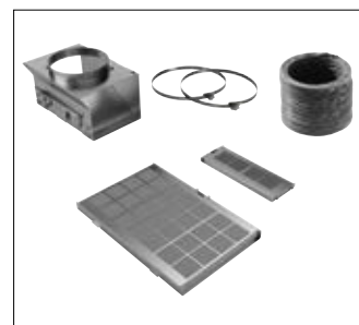
DWZ 0AK0S0: zestaw startowy do pracy w obiegu zamkniętym do regeneracji. Zawiera zwrotnicę do pracy w obiegu zamkniętym, filtr z aktywnym węglem do wielokrotnej regeneracji (2 szt.), elastyczny wąż i materiał do mocowania.
