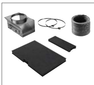
DWZ 0AK0U0: zestaw startowy do pracy w obiegu zamkniętym. Zawiera zwrotnicę do pracy w obiegu zamkniętym, filtr z aktywnym węglem (2 szt.), elastyczny wąż i materiał do mocowania.
