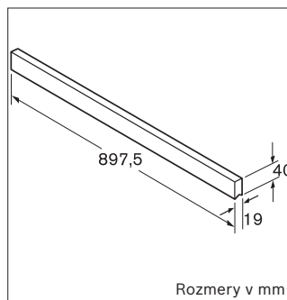
DHZ 4950
