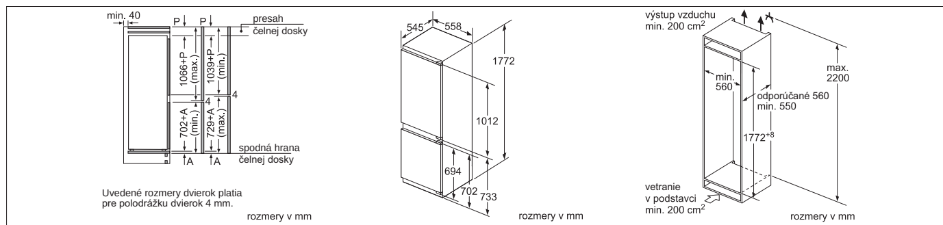
KIS 86AF30
