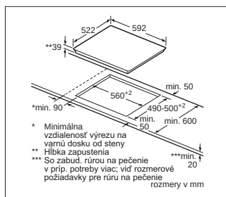
PKE611B17E | PKN651FP1E
