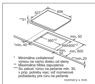
PXE675DC1E
