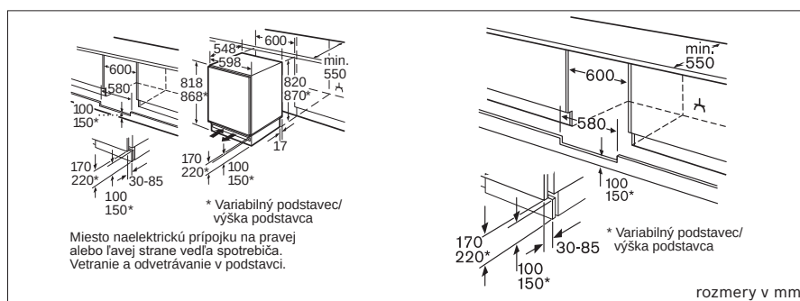
KUL 15A65
