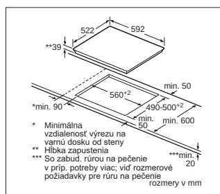
PKF651B17E | PKF659C17E
