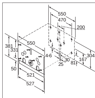
DSZ 4960 | DSZ 4660
