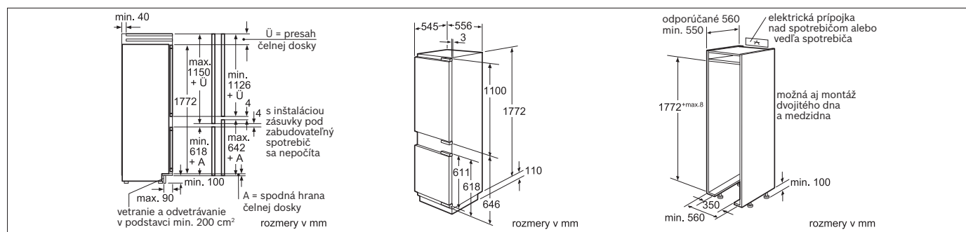
KIF 39S80
