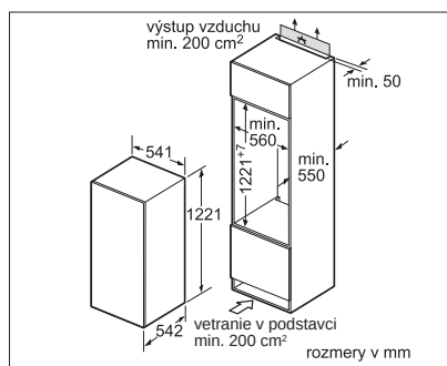
KIL 24V21FF
