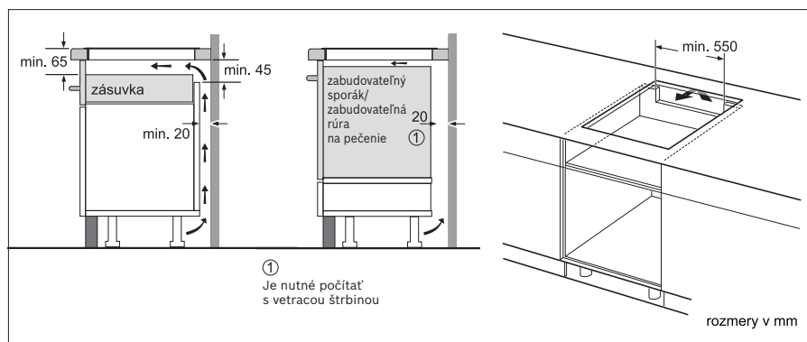
PKE611B17E | PKN651FP1E
