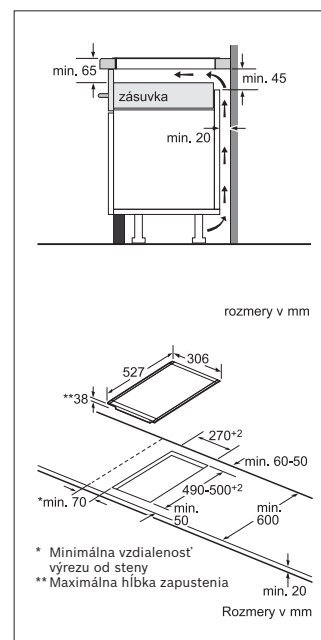
PKF375FP1E
