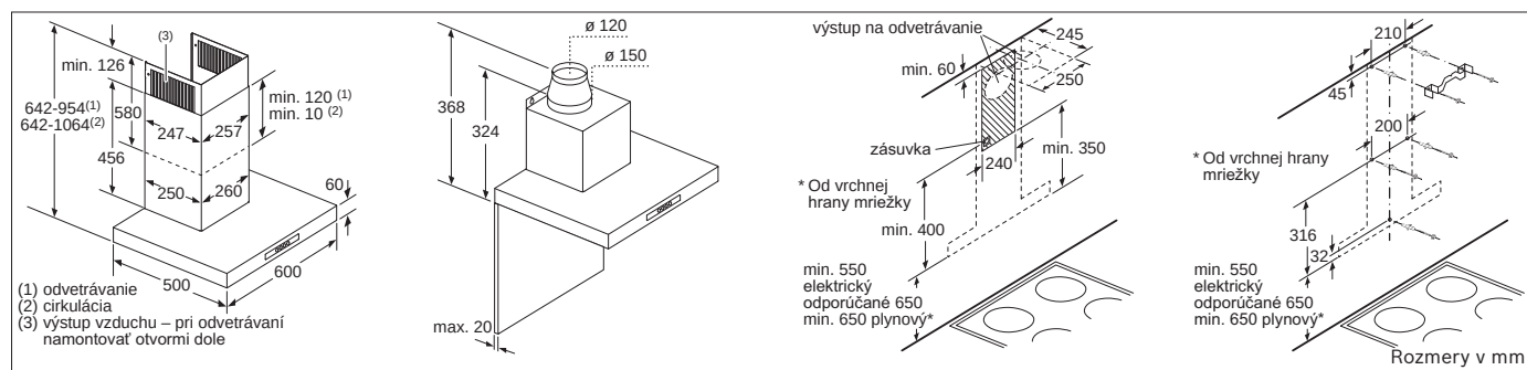
DWB 06W452
