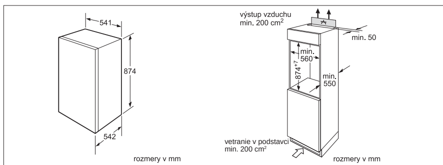
KIL 18V60
