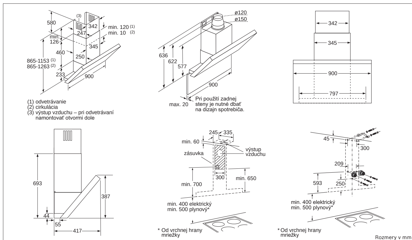
DWK 098E50
