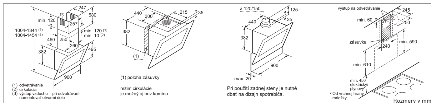
DWK 098G1
