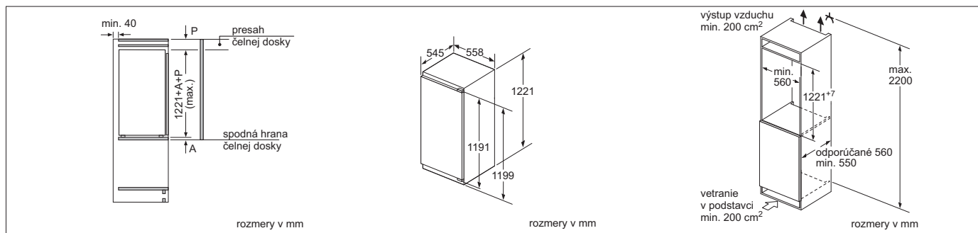
KIF 42AF30
