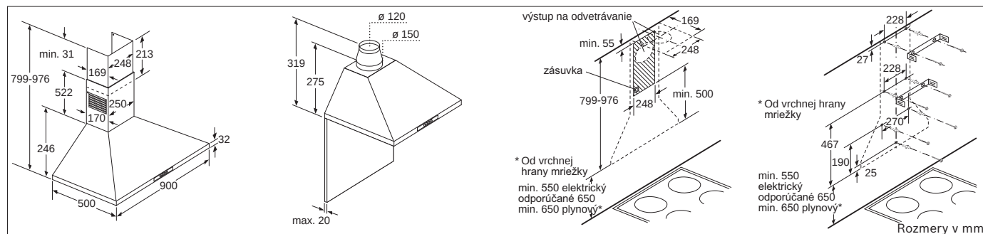
DWW 09W450
