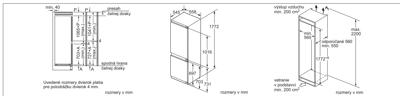
KIS 86AD40
