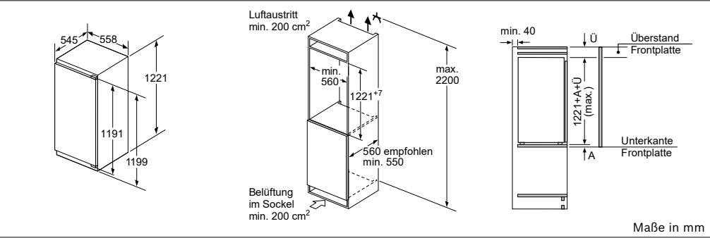
KIF 41SD30 | KIF 42SD30 | KIR 41SD30 | KIL 42SD30 | KIF41SD40 | KIR 41SD40
