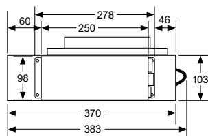
Ansicht Steuereinheit
