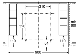
Montage Gerät mit Absenkrahmen Möbel mit seitlichen Regalfächern Montage direkt an der Küchenwand
