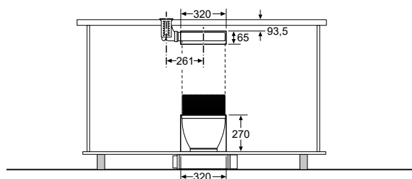
Ausschnitt in Rückwand
