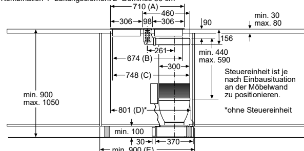
Kombination 2×Lüftungselemente 3×Dominos 30 cm
