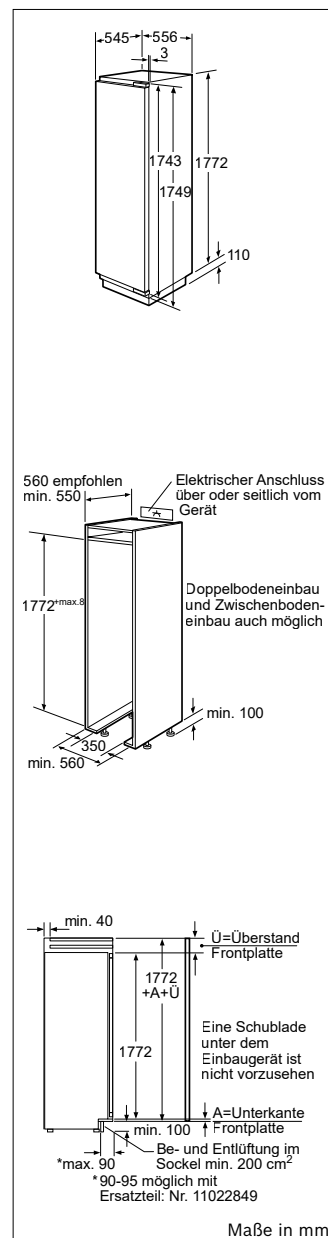
KIF 42S80 | KIF 40S80
