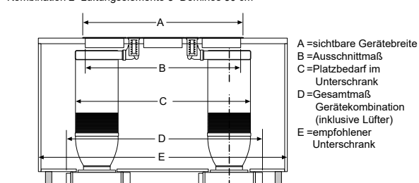
Kombination 2×Lüftungselemente 3×Dominos 30 cm
