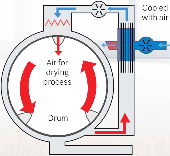
Drying motor fan
