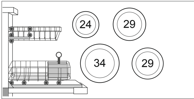
Korbsystem ohne VarioSchublade, Gerätehöhe 86,5 cm (Der 5 cm höhere Geschirrspüler schafft Raum für hohe Geschirrtteile im Unterkorb.)
