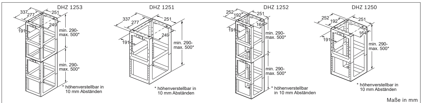
Montageturmverlängerungen DHZ 1253 | 1251 | 1252 | 1250
