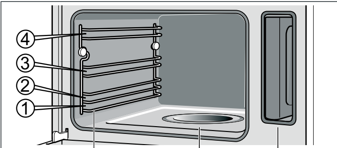
Gestelle für das Zubehör Verdampferschale Tankschacht mit Wassertank
