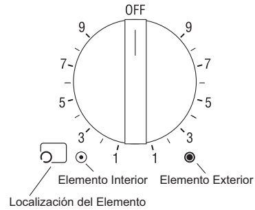
Figura 9: Perilla de control de un elemento doble
