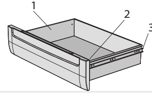
Figure 12: Pièces du tiroir réchaud
