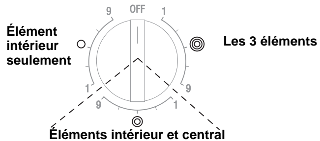
Figure 10: Bouton pour élément triple
