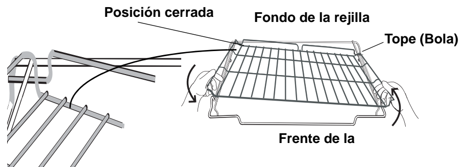
Figura 5: Reensamblado
