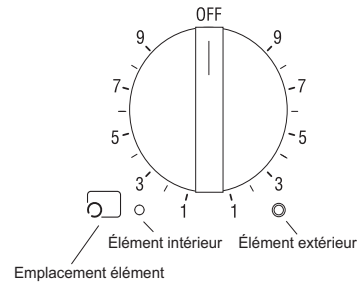
Figure 9: Bouton de contrôle d'élément jumelé
