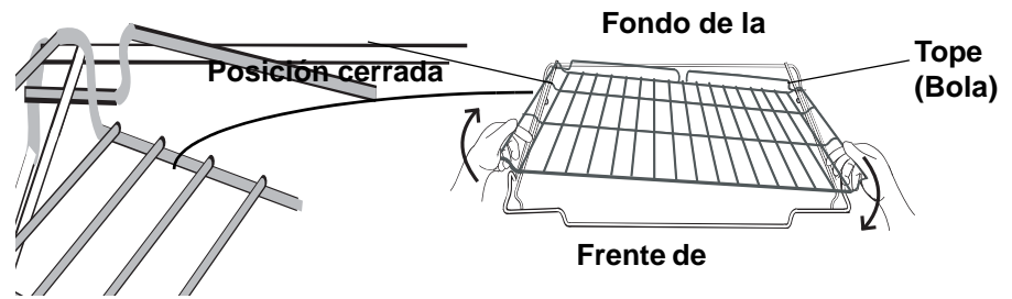
Figura 4: Desmontaje
