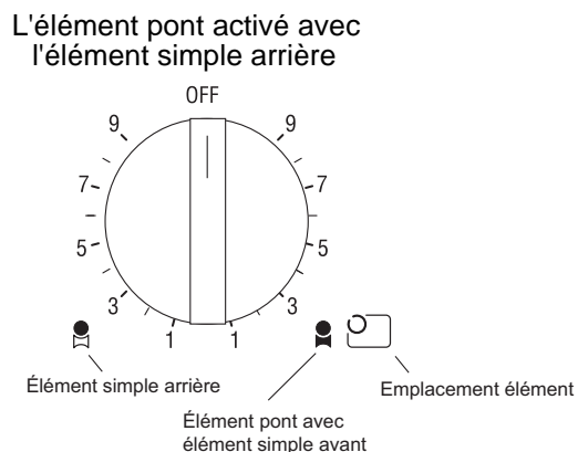
Figure 11: Bouton d'élément pon
