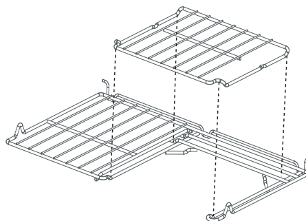
Figura 6: Rejilla media del horno
