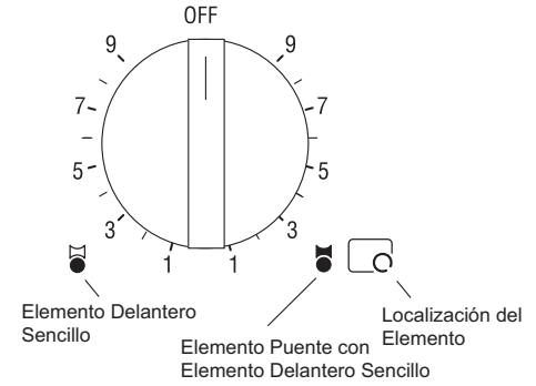
Figure 11: Perilla de control del elemento puente
