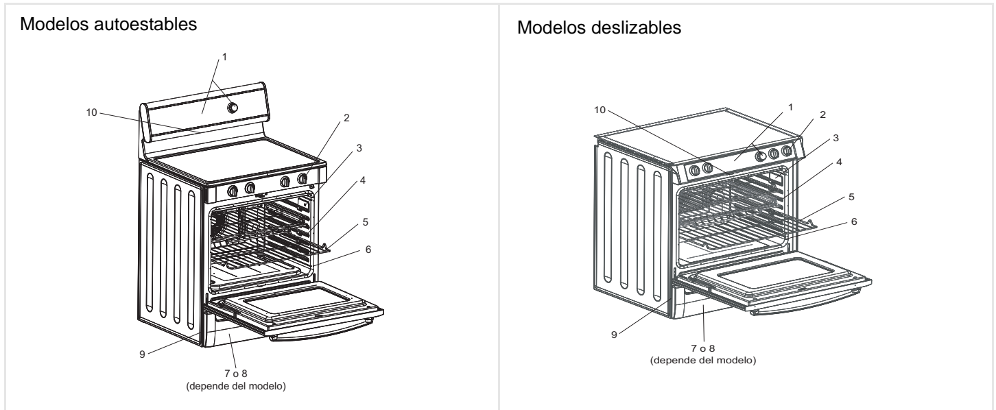
Figura 1: Partes y accesorios
