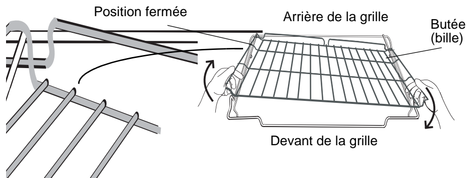
Figure 4: Démontage
