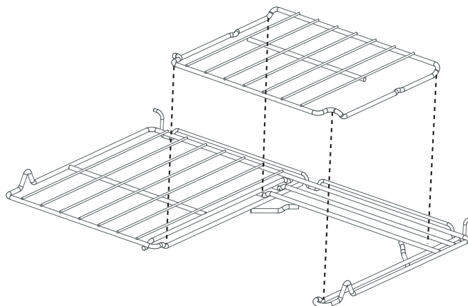
Figura 11: Rejilla media del horno
