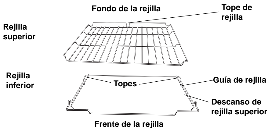
Figura 8: Rejilla de extensión completa
