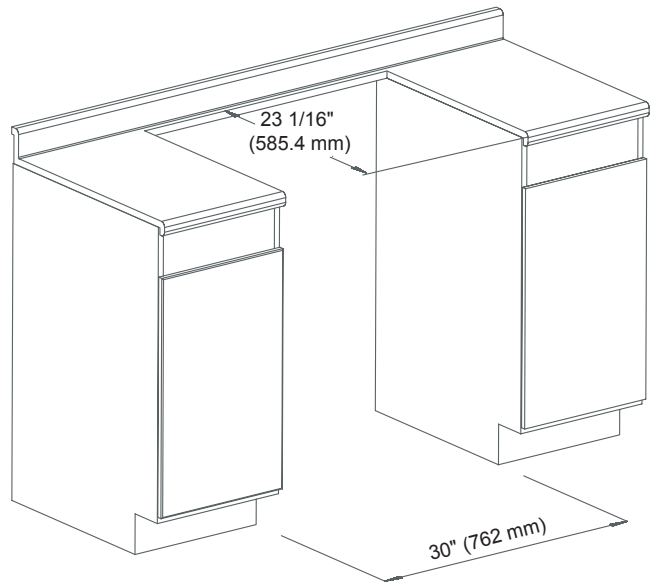
Figura 2: Requerimientos del recorte
