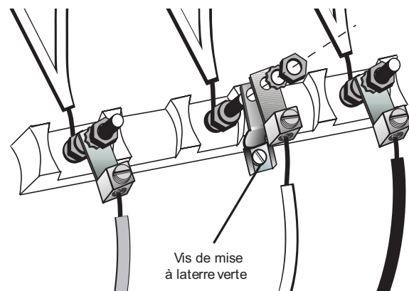
Figure 22: Conduit flexible à 3 fil complété
