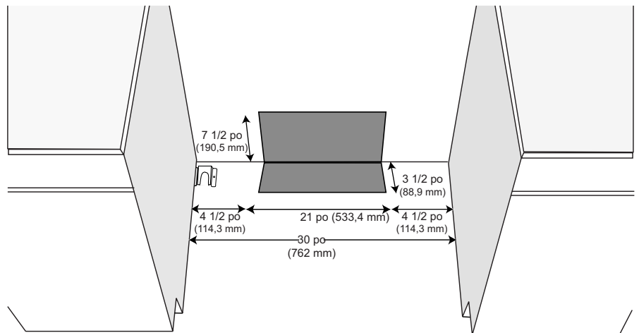
Figure 1: Dégageements de la surface de cuisson
