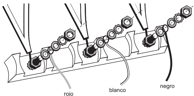
Figura 12: Conexión del cable de 4 hilos, continuación
