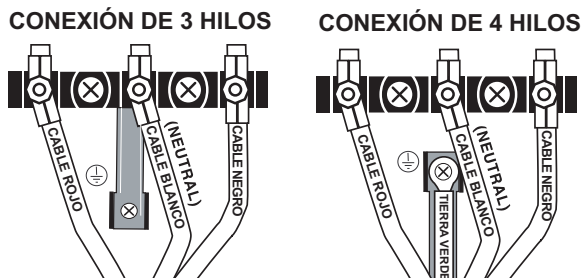
Figura 9: Requerimientos para la puesta a tierra
