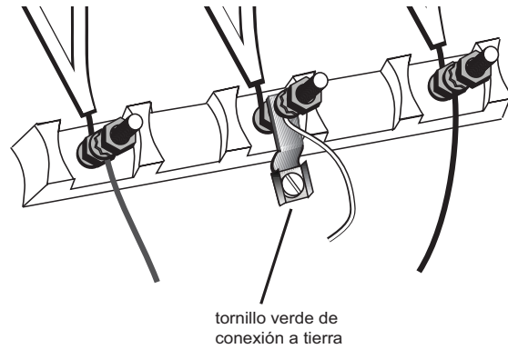
Figura 15: Conexión terminada del cable de la estufa de 3 hilos
