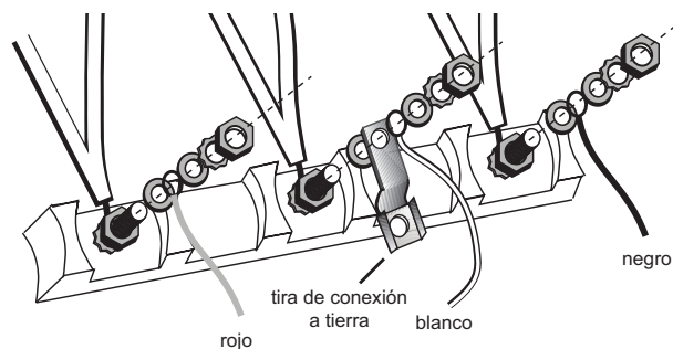
Figura 14: Conexión de 3 hilos
