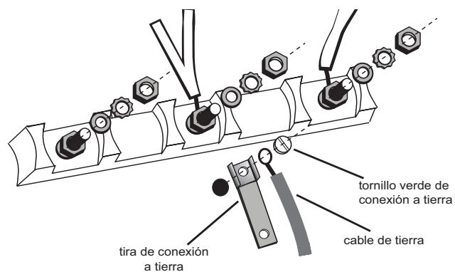
Figura 11: Conexión del cable de 4 hilos - Tira y cable de tierra
