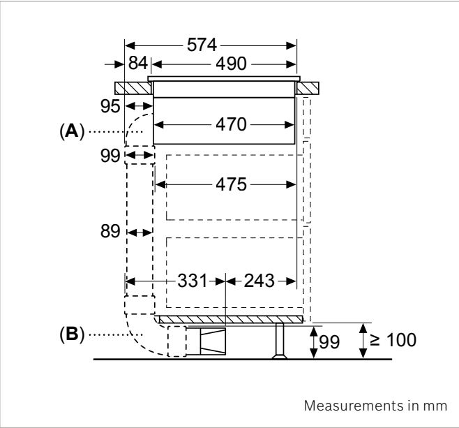
PVQ731F15E/PVQ811F15E
