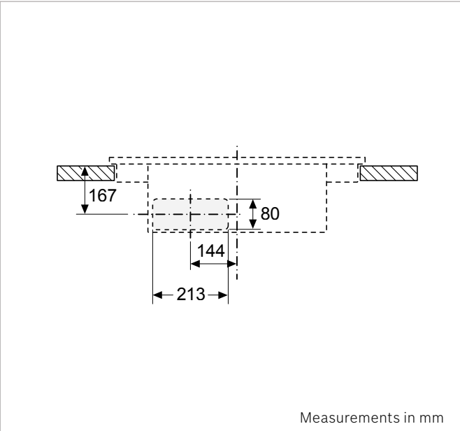
PVQ731F15E/PVQ811F15E
