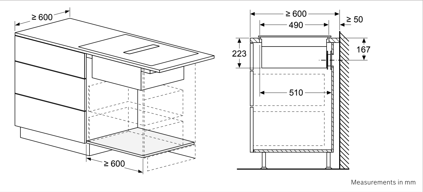
PVQ731F15E/PVQ811F15E
