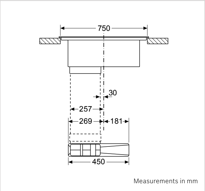
PVQ811F15E
