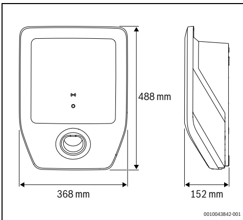
Fig. 388 Dimensões do produto
