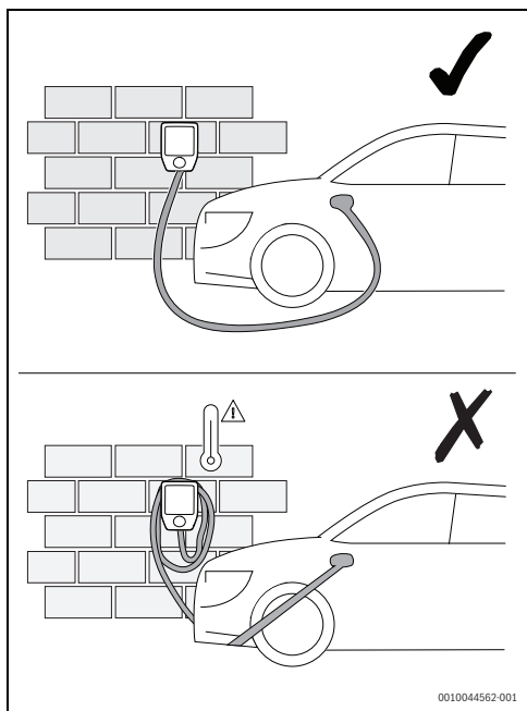
Rys. 382 Postępowanie z kablem ładowania
