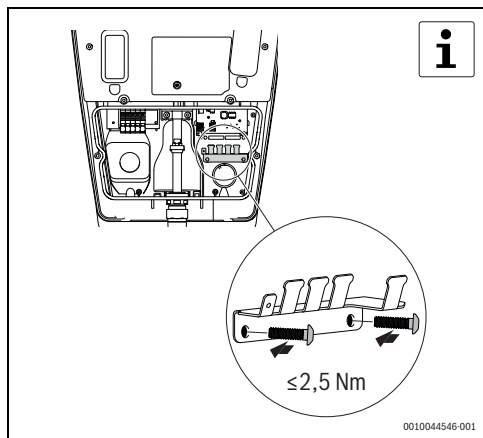
Sl.471 Namestitev držala za kabel
