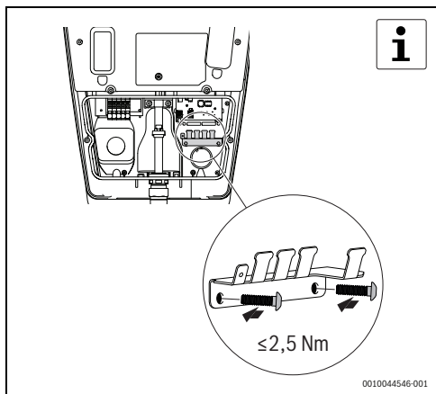
255. ábra A kábeltartó felszerelése
