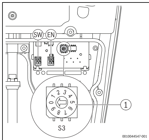
Fig. 206 Bouton de sélection du courant max. (S3)
