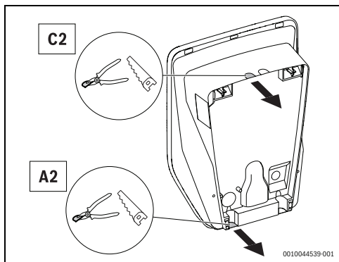
Fig. 106 Dækslet på eltilslutninger
