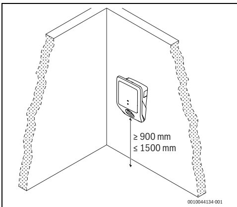
Afb. 293 Minimale afstanden
