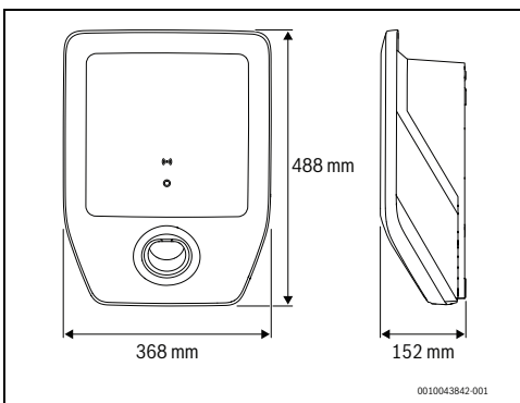
Afb. 292 Productafmetingen
